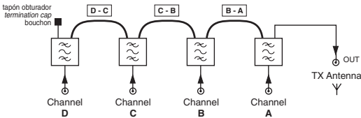
Diagrama de Bloques del XRA-400 para 4 Canales Block Diagram of the XRA-400 for 4 Channels Schéma Synoptique du XRA-400 pour 4 Canaux
